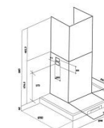
Schéma d'encastrement
