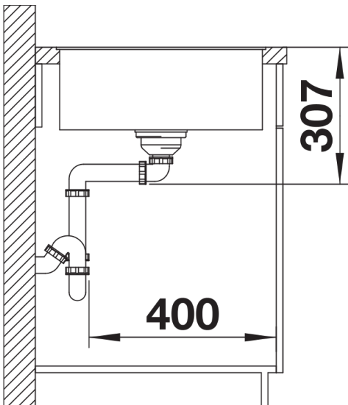
Vue latérale
