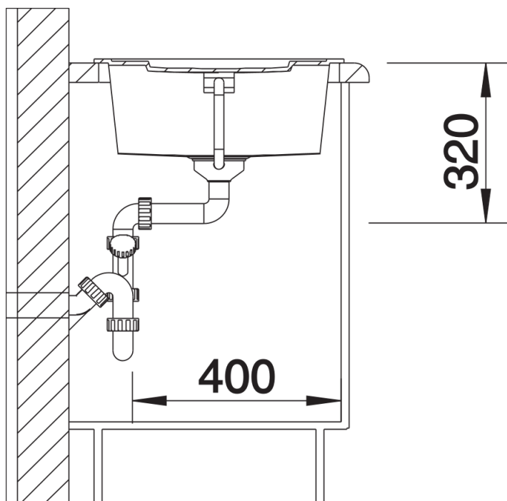
Vue latérale
